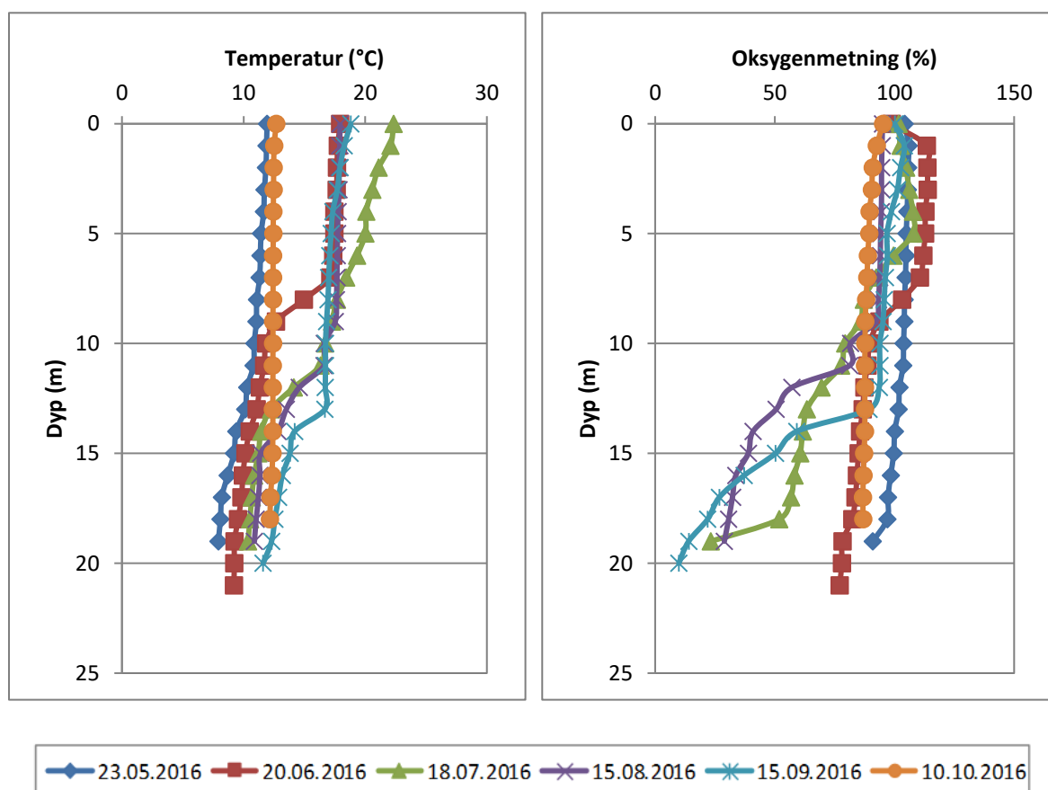
Fig. 1 Temperaturprofiler og oksygenprofiler fra Steinsfjorden i 2016
