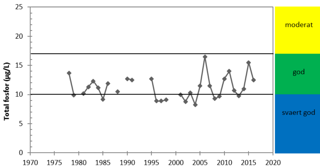
Fig. 2 Fosforkonsentrasjonen i Steinsfjorden (0-7 m dyp) for perioden 1978-2016. Figuren viser middelveidien av total fosfor for hvert års vekstsesong (mai-oktober). Grensene mellom de ulike økologiske tilstandsklassene er også vist. Miljømålet er grensen mellom tilstandsklassene god og moderat.
